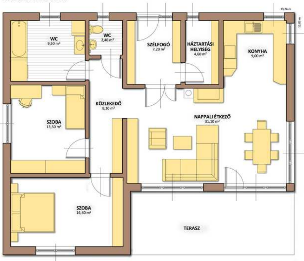
FÖLDSZINTI ALAPRAJZ
